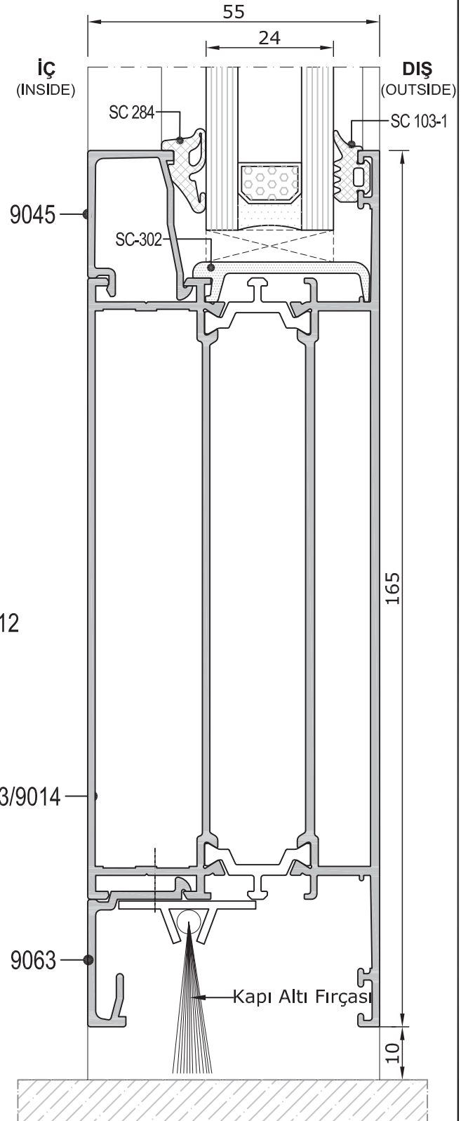
Inside or Outside Openning Flat Door System Detail İçe veya Dışa Açılır Hemyüz Kapı Sistem Detayı
