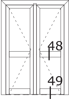
Inside or Outside Openning Flat Door System Detail İçe veya Dışa Açılır Hemyüz Kapı Sistem Detayı
