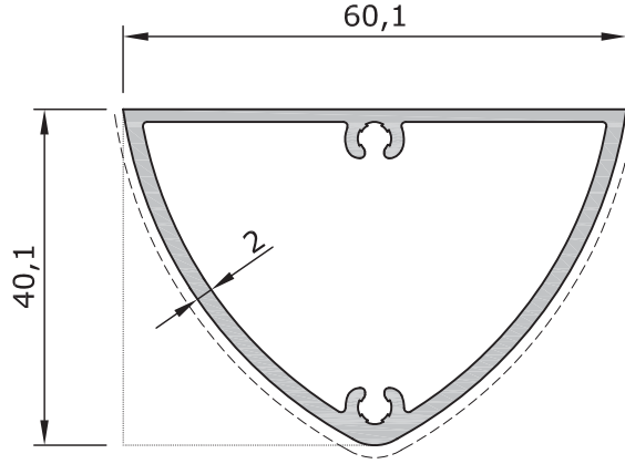
9142** | Orta Kayıt Takviye Profili 0,865 kg/m | Reinforced Profile for Transom J_x=6,07 \text{ cm}^4 | J_y=9,66 \text{ cm}^4
