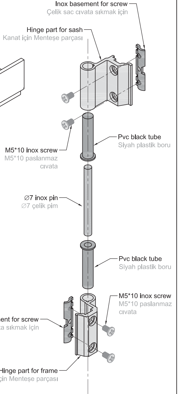
EXPLODED VIEW of HINGE PARÇA YERLEŞİM GÖRÜNÜŞÜ
